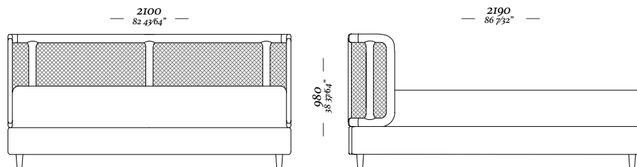
CAMA MONTADA 193
