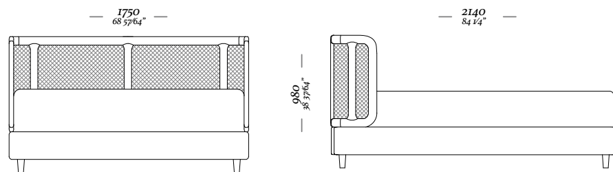
CAMA MONTADA 158
