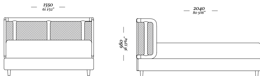
CAMA MONTADA 138
